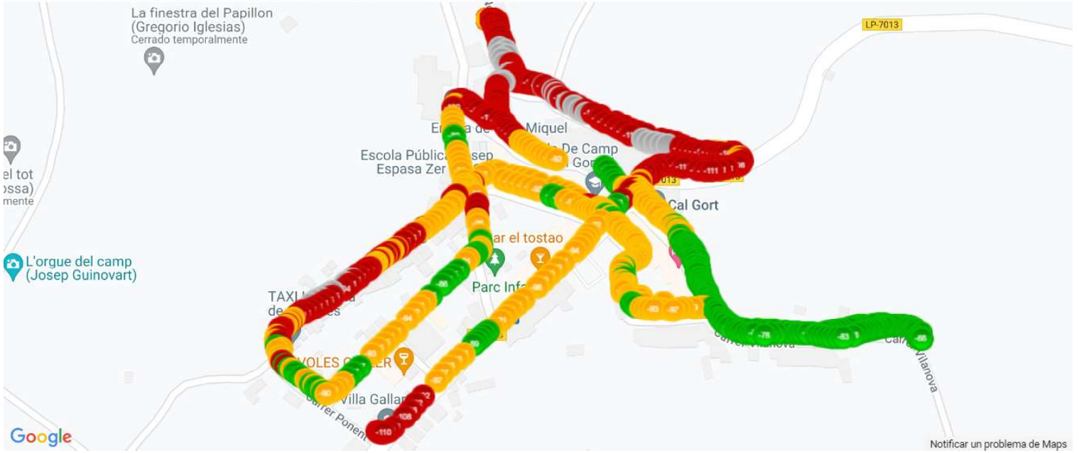
MOVISTAR SERVEI DE DADES, MAPA DE NIVELL DE SENYAL, LA POBLA DE CÉRVOLES
