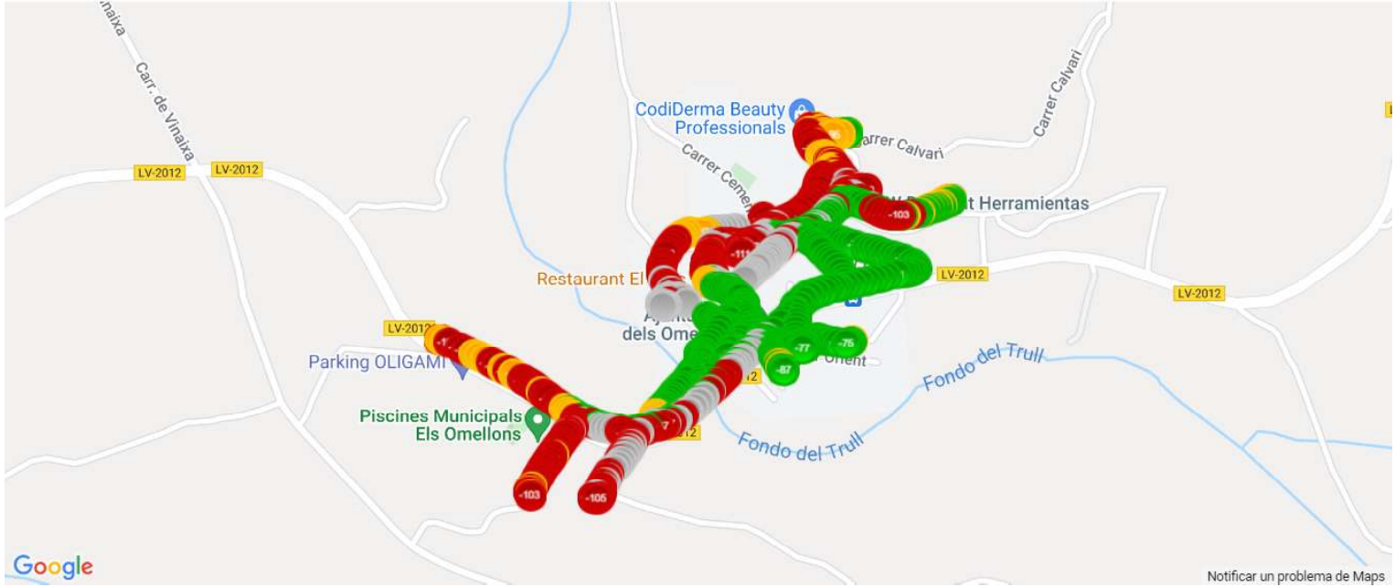
ORANGE SERVEI DE DADES, MAPA DE NIVELL DE SENYAL, ELS OMELLONS
