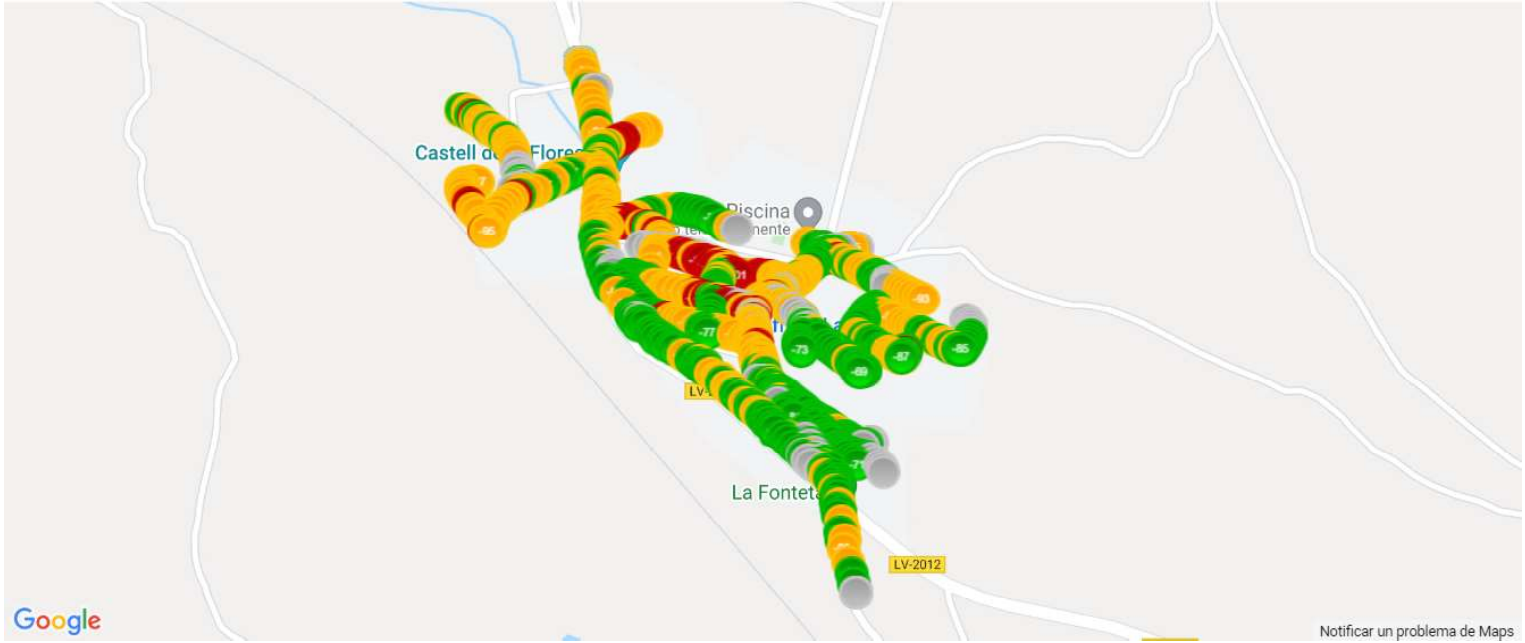
MOVISTAR SERVEI DE VEU, MAPA DE NIVELL DE SENYAL, LA FLORESTA
