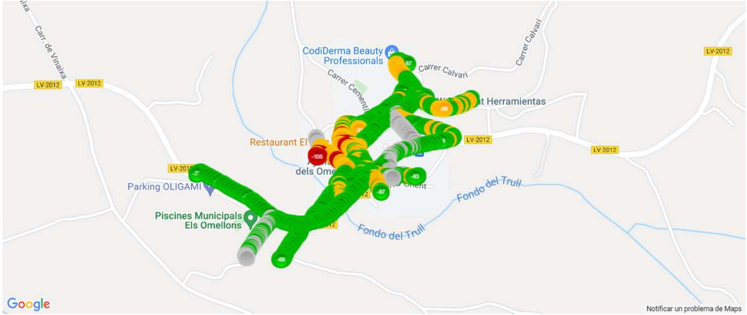
MOVISTAR SERVEI DE DADES, MAPA DE NIVELL DE SENYAL 3G, ELS OMELLONS
