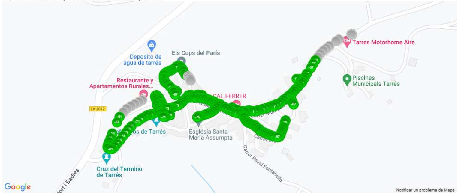
ORANGE SERVEI DE VEU, MAPA DE NIVELL DE SENYAL, TARRÉS
